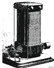
Dynamo z počátku 20. století. Svými parametry (stejnoseměrný proud asi 10 A o napětí 50 V) bylo určeno pro využití v domácnosti.
