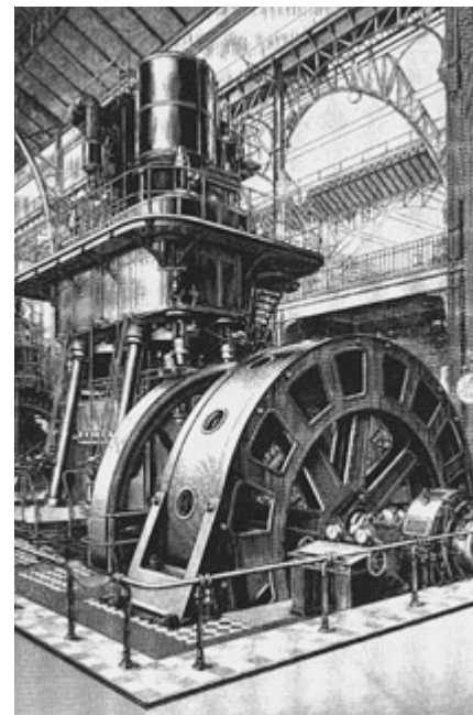
Obrovské dynamo poháněné mohutným parním strojem, které bylo vyrobeno Siemensovou továrnou
