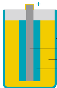
Suchý Leclanchéův článek
