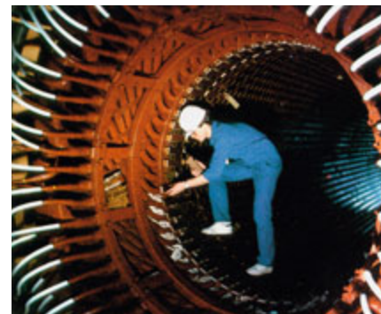
Stator turboalternátoru při montáži
