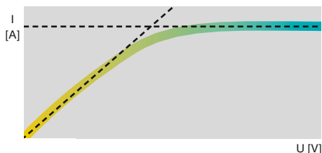
Nesamostatný výboj v plynech
