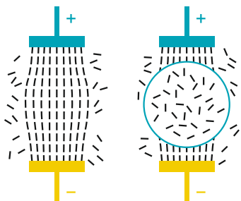
Siločáry v rovině a efekt stínění elektrického pole
