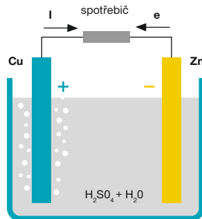
Princip galvanického článku
