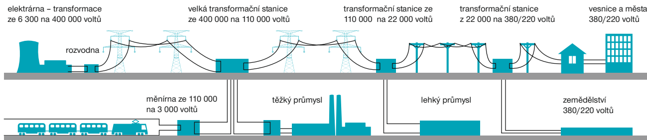
Propojení výroby a spotřeby elektrické energie
