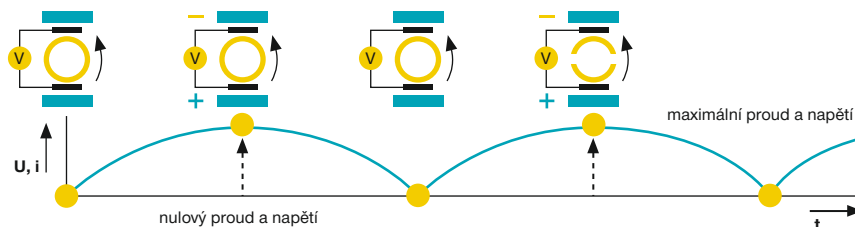
Činnost komutátoru dynama
