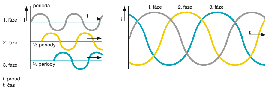
Graf třífázového proudu
