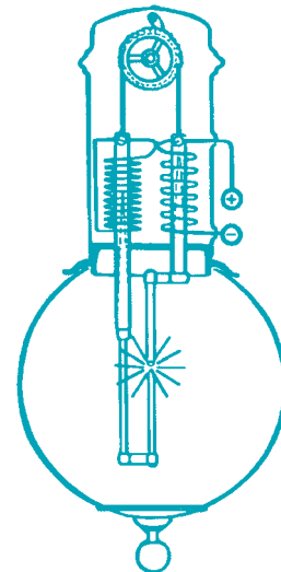
Princip Křížíkovy obloukové lampy
