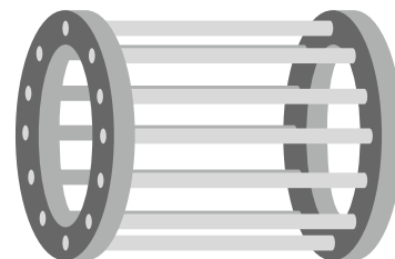
Vinutí rotoru asynchronního stroje nakrátko (někdy se nazývá klecové vinutí)
