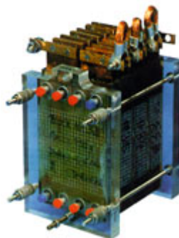
Olověné desky průmyslového akumulátoru s kapacitou 400 W
