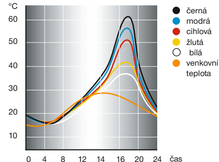
Denní průběh teploty povrchů
