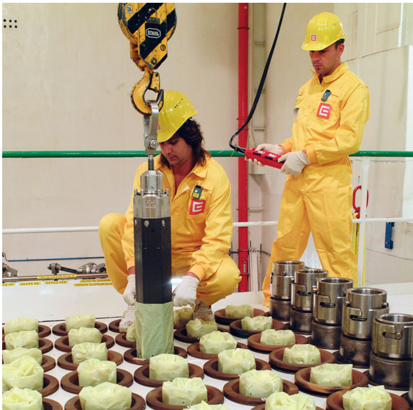
Sklad čerstvého paliva v Jaderné elektrárně Dukovany
