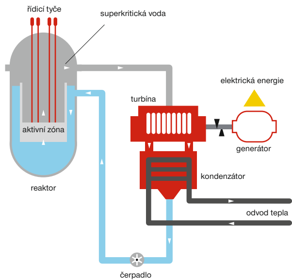
Schéma uspořádání superkritickou vodou chlazeného reaktorového systému
