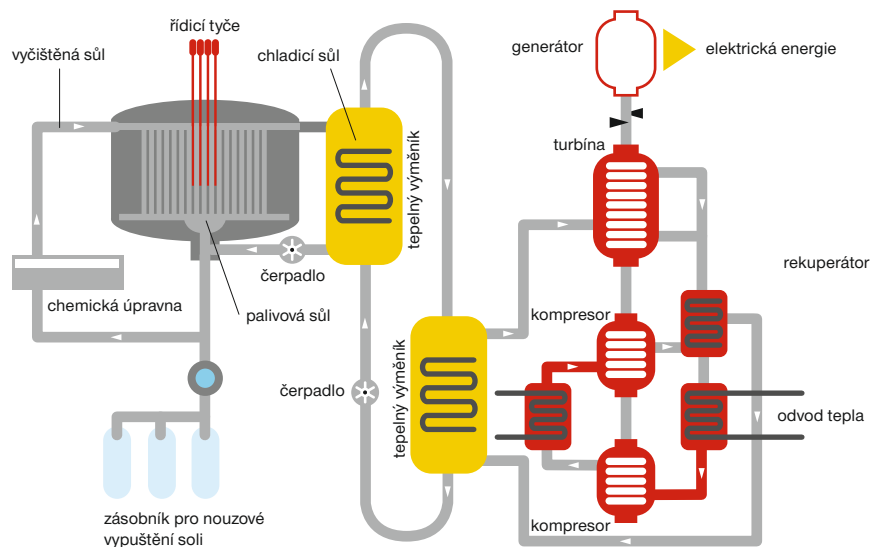
Schéma uspořádání reaktorového systému s roztavenými solemi
