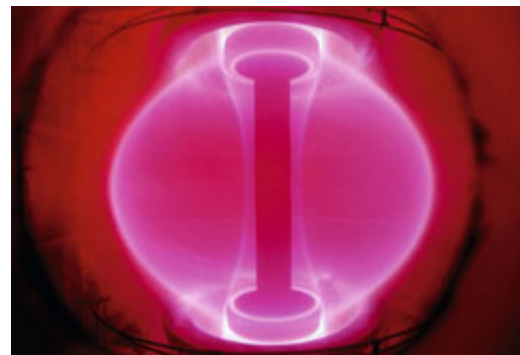
Pohled do nitra tokamaku na žhavé plazma
