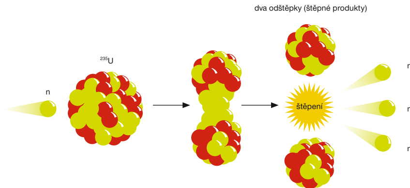
Princip štěpné řetězové reakce
