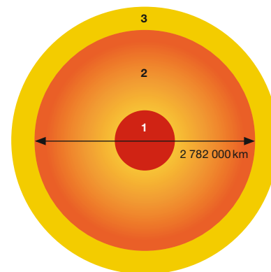
Průřez Sluncem: (1) aktivní oblast kolem slunečního středu, ve které probíhají termonukleární reakce; (2) vrstva horké sluneční hmoty, která tvoří izolaci aktivní oblasti; (3) sluneční atmosféra
