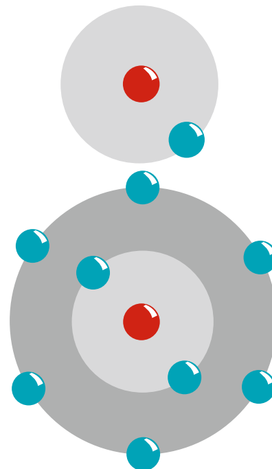
Modely atomu vodíku a kyslíku
