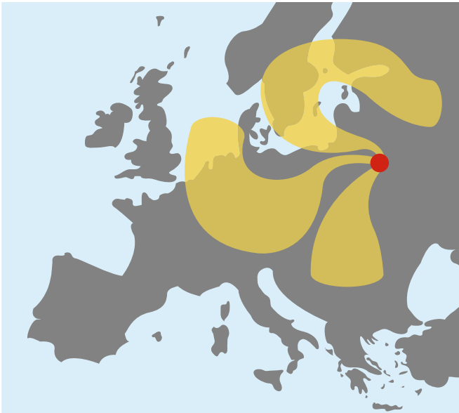
Radioaktivní mračno v prvních třech dnech po havárii
