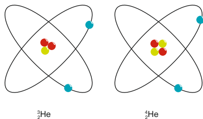
Izotopy helia
