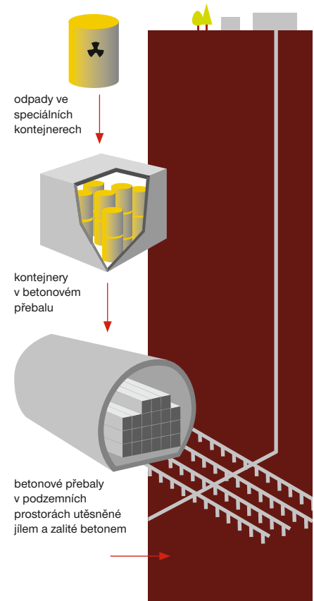
Schéma ukládání opadu do hlubinného úložiště – bezpečnostní bariéry
