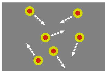
B ●● atom deuteria
