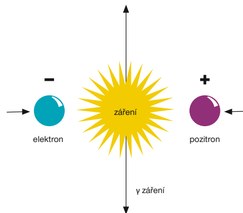
Schéma anihilace – částice elektron se svou antičásticí pozitronem. Setkají-li se částice s antičásticí, dojde k anihilaci, při které se uvolní jejich klidová energie a změní se v příslušné množství záření. Využití klidové energie je až 100 %.
