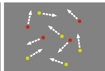
C ● deutron ● elektron
