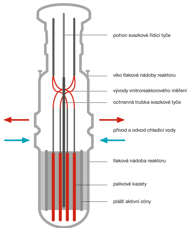
Schéma tlakovodního jaderného reaktoru
