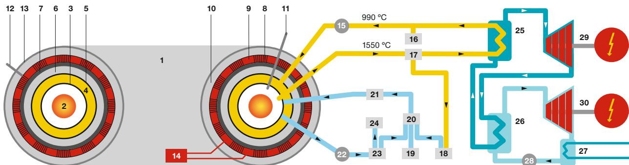
Celkové energetické schéma termonukleárního fúzního reaktoru
